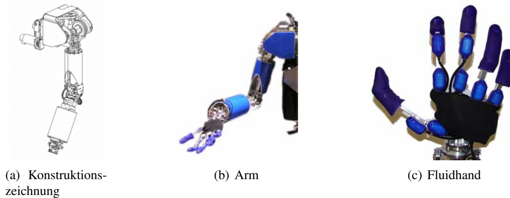
Abb. 5.7.: Konstruktionszeichnung des Arms. Aufnahme des Arms mit den haptischen Sensoren auf der Schulter und am Ober- und Unterarm. Aufnahme der Fluidhand in der mit Druckluft betriebenen Variante.
