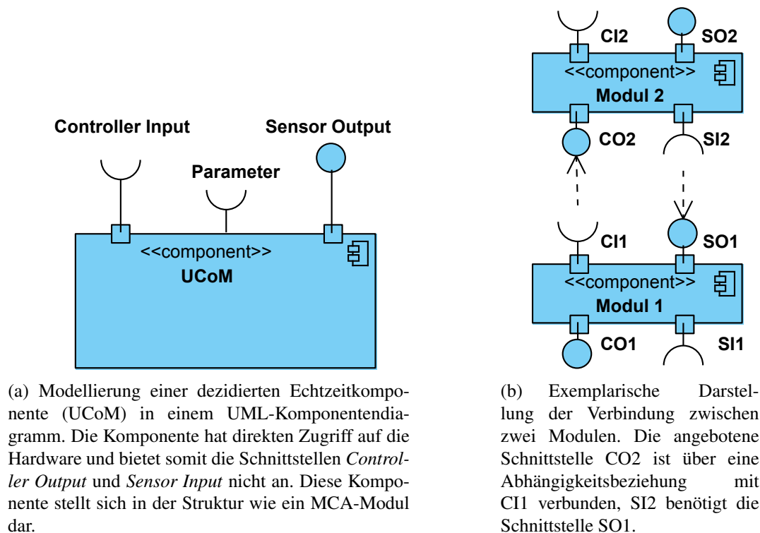
Abb. 4.8.: Dezidierte Echtzeitkomponente (UCoM) als MCA-Modul und formale Darstellung der Verbindung zwischen zwei Modulen
