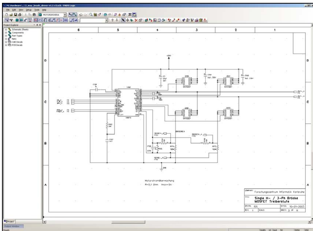
Abb. D.1.: Screenshot der zum Schaltplanentwurf verwendeten Software PADS Logic. Es ist ein Ausschnitt aus dem Schaltplan des Dreier-Motorboards – die Beschaltung eines H-Brückentreibers zur Motoransteuerung – dargestellt.
