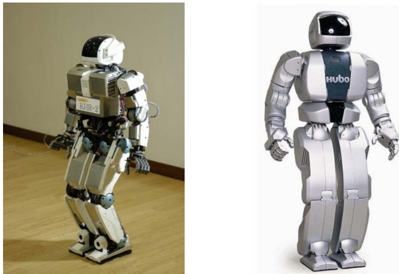
Abb. 2.18.: Die humanoiden Roboter KHR-2 (links) und KHR-3/HUBO (rechts)
