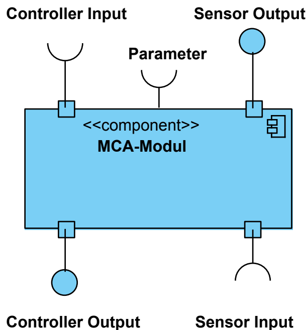
Abb. 4.6.: Modellierung eines MCA-Moduls als Komponente in einem UML-Komponentendiagramm
