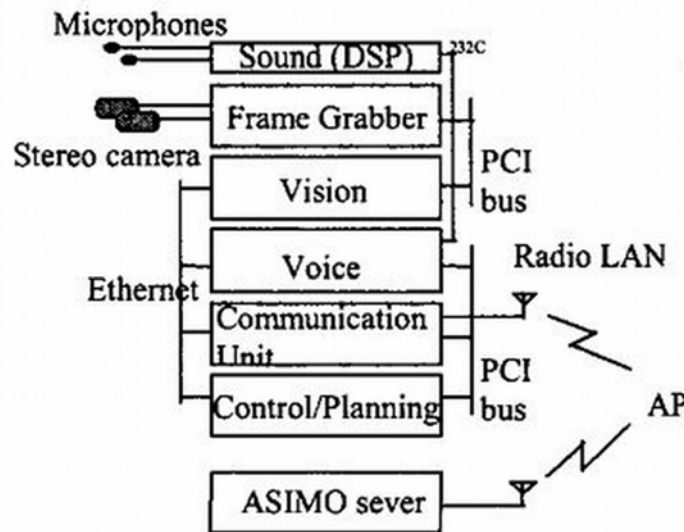
Abb. 2.12.: Der humanoide Roboter ASIMO und die verwendete Architektur [134]
