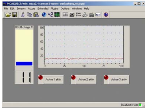
(a) Die Grundaustlastung des UCoMs liegt für 1 ms Zykluszeit bei circa 10%
