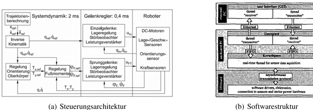
Abb. 2.22.: Steuerungsarchitektur und Softwarestruktur auf JOHNNIE (Quelle: [151, 103])
