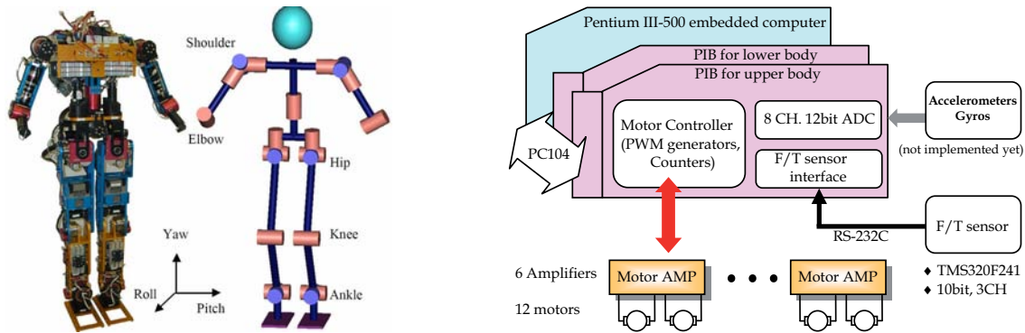
Abb. 2.17.: Der humanoide Roboter KHR und die verwendete Rechnerarchitektur (Quelle [93])
