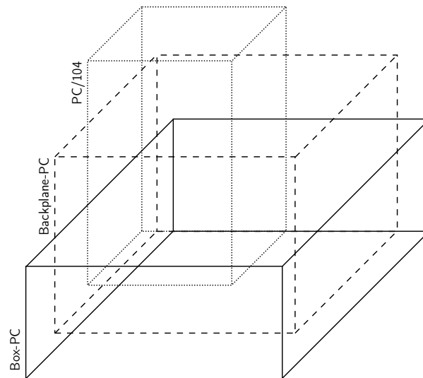
Abb. 4.12.: Vergleich der unterschiedlichen Formfaktoren von Recheneinheiten. Die Außenmaße der jeweiligen Rechnertypen sind als Quader dargestellt. Die Abmessungen des Backplane-PCs sind mit gestrichelten, die des PC/104 mit gepunkteten und die des Box-PCs mit durchgezogenen Linien eingezeichnet.
