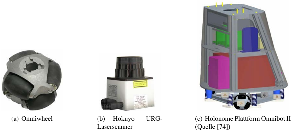
Abb. 5.4.: Das für den Antrieb der Plattform verwendete Omniwheel, der Hokuyo URG-Laserscanner zur Erfassung der Position der Plattform anhand einer gespeicherten Karte und die Konstruktionszeichnung der holonomen Plattform
