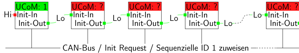
(b) Bootloader setzt alle Init-Ausgänge auf Lo, Nummer 1 wird zugewiesen
