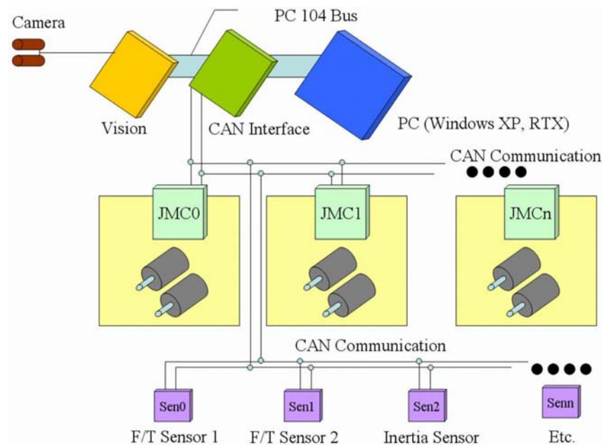
Abb. 2.19.: Rechnerarchitektur im humanoiden Roboter KHR-2 (Quelle [119])
