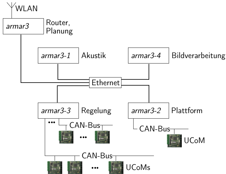
Abb. 5.8.: Struktur der verteilten Systemarchitektur auf ARMAR-III. Die Verteilung auf die Recheneinheiten erfolgt anforderungsbezogen und nach Domänen gruppiert. armar3-3 und die UCoMs stellen den echtzeitfähigen Teil bereit.
