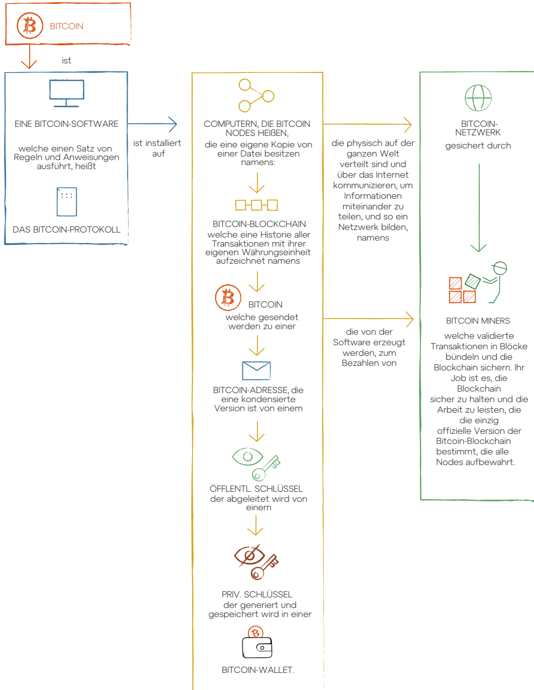
ABBILDUNG 55: DAS BITCOIN-SYSTEM
