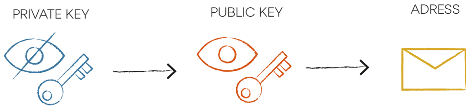
ABBILDUNG 43: EINWEGFUNKTION
